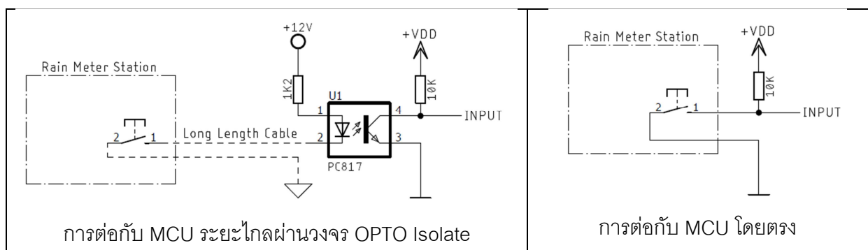
ตัวอย่าง การเชื่อมต่อกับไมโครคอนโทรลเลอร์
